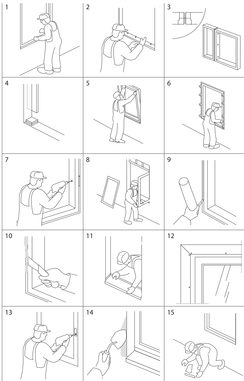
Fönstermonterings olika skeden (RT 103241)
